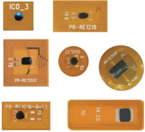
FPCB RFID Tag
